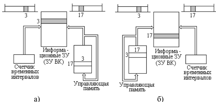
Рис. 9 Способы работы временного коммутатора:
