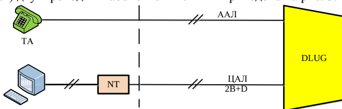
Рис. 3 – Схема подключения аналоговых и цифровых АЛ (ТА – аналоговый телефонный аппарат, ТЕ – цифровой абонентский терминал ISDN, NT – сетевое окончание ISDN)
