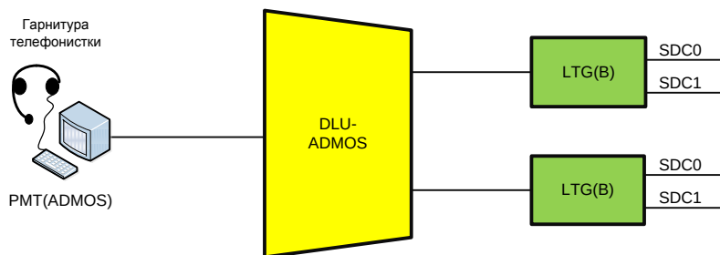
Рис. 9 - Схема подключения рабочих мест телефонисток
