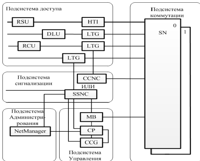
Рис. 1 - Основные функциональные подсистемы EWSD
