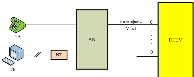
Рис. 8 - Схема подключения AN через DLUV
