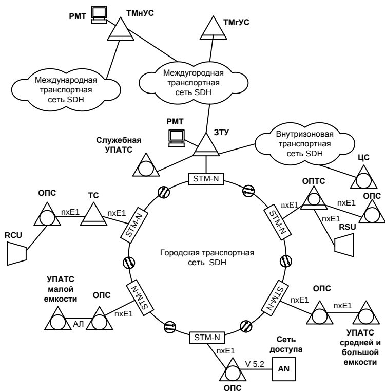
Рис. 2 – Схема возможных применений системы EWSD на сети связи
