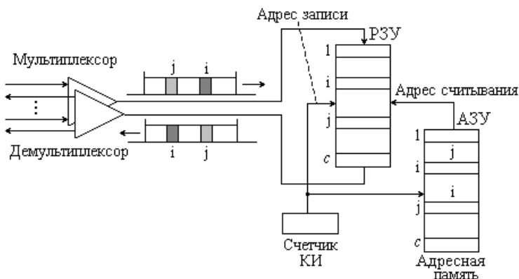
Рис. 8 - Структурная схема временного коммутатора
