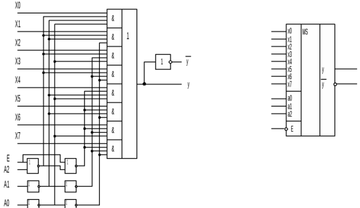
Рис. 3 - Мультиплексор на 8 входов: логическая схема и обозначение
