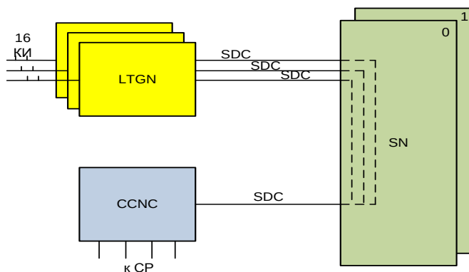
Рис. 10 – Схема подключения звеньев ОКС №7
