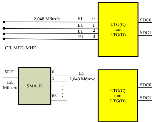
Рис. 7 – Схема подключения цифровых СЛ и групповых трактов SDH
