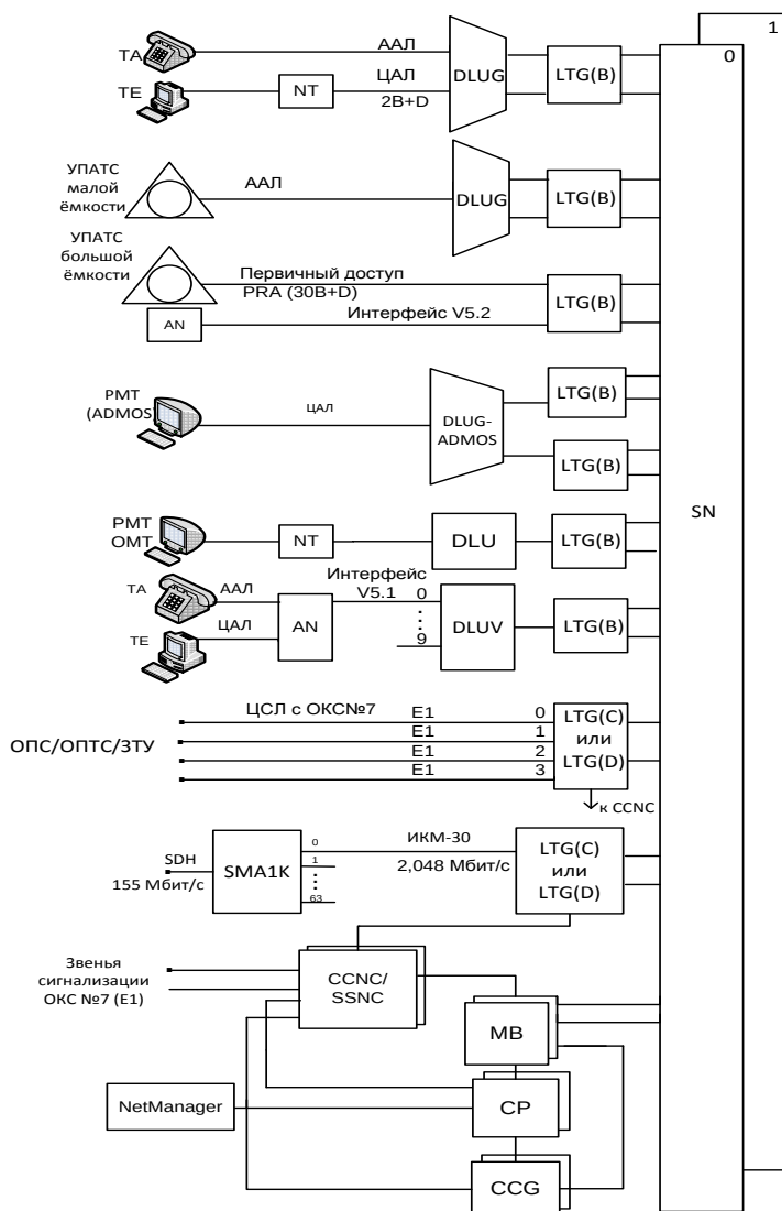
Рис. 12 Пример структурной схемы системы EWSD
