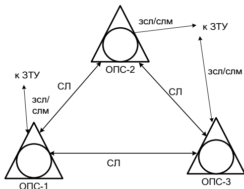
Рис. 3 – Районированная ГТС
