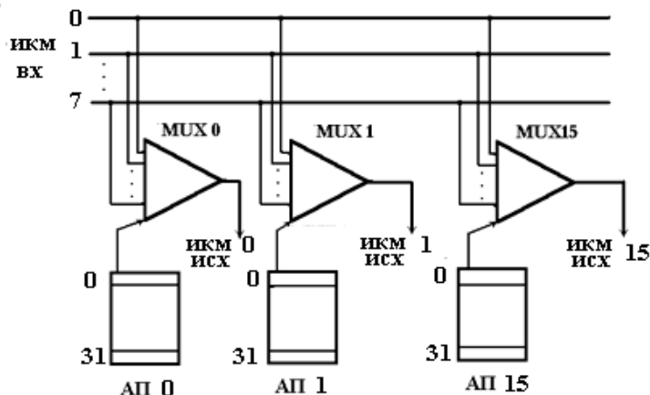
Рис. 5 - Схема пространственного коммутатора 8х16 на мультиплексорах
