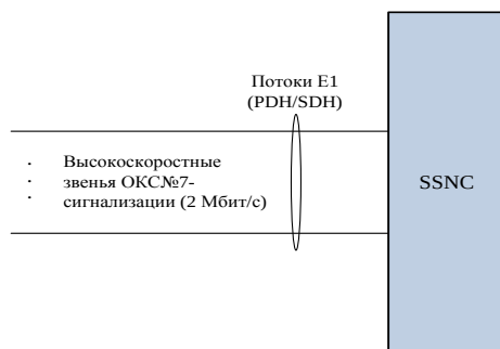
Рис. 11 – Схема подключения звеньев сигнализации ОК №7 со скоростью 2 Мбит/с
